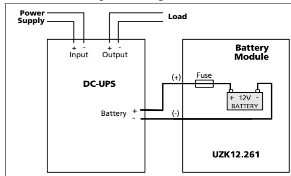
Fig. 8-1 Wiring scheme
