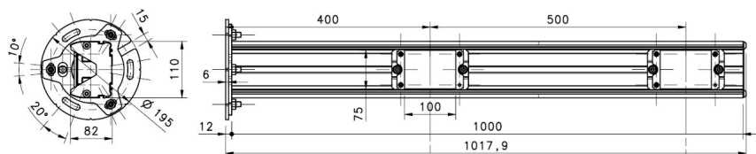
SG-PSM-3-800
