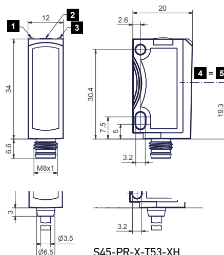
S45-PR-X-T53-XH S45-PR-X-B53-XH
