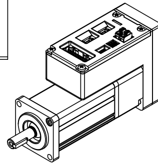
MDXR42JNBRC A000 尺寸图 MDXR42JNBRC A000 2D drawing
