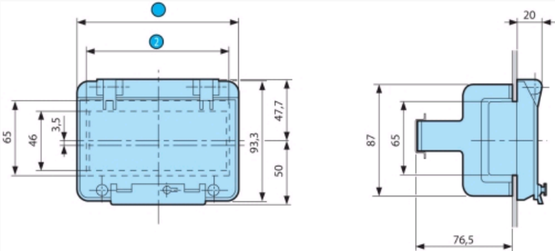
Dimension Diagram : IP67
