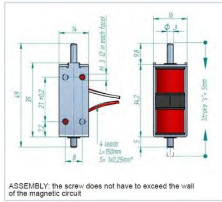
Dimensionnal drawing:
