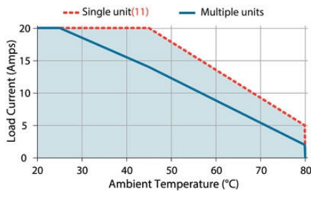
DR2260x20x
