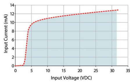
4-32 VDC Input
