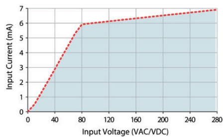
90-280 VAC/VDC Input
