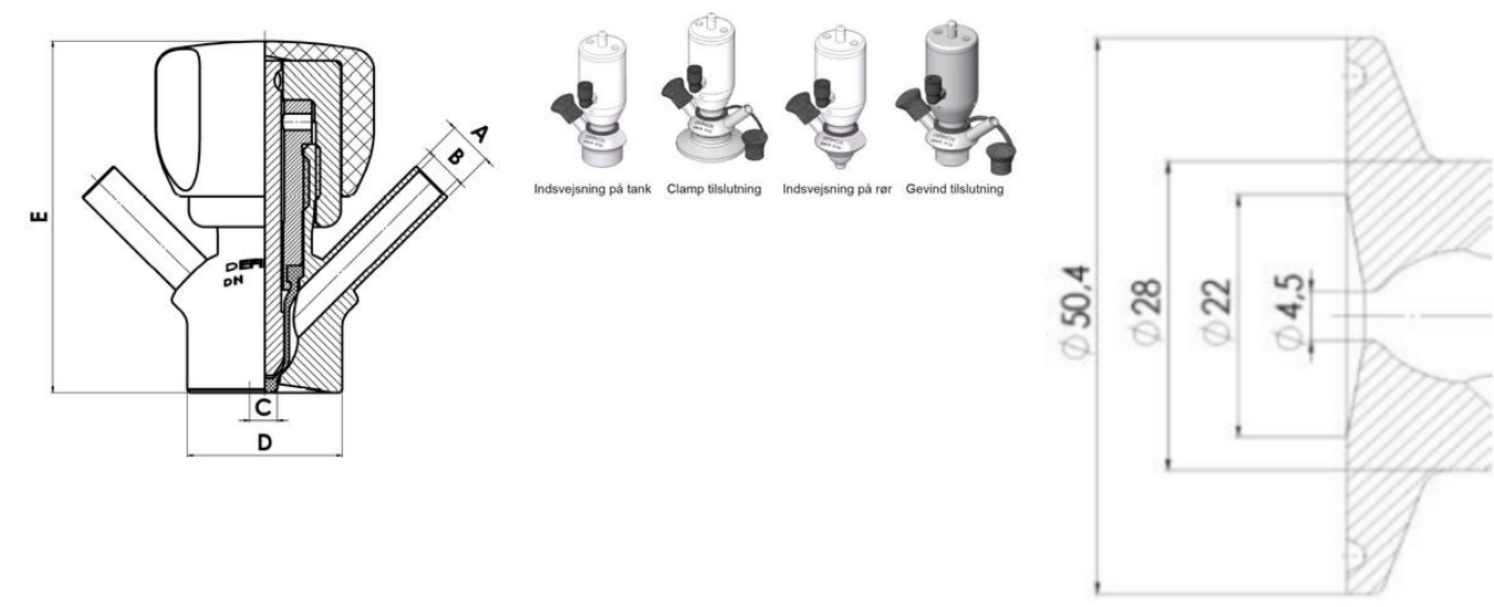
Clamp Ø 50,4
