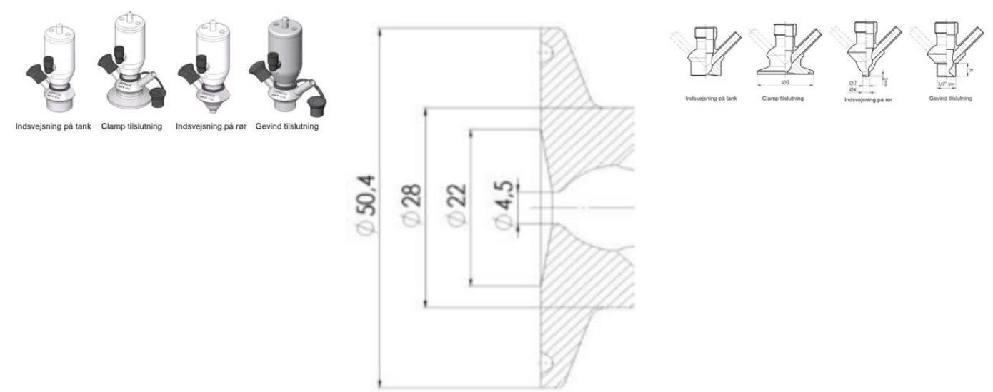
Clamp Ø 50,4
