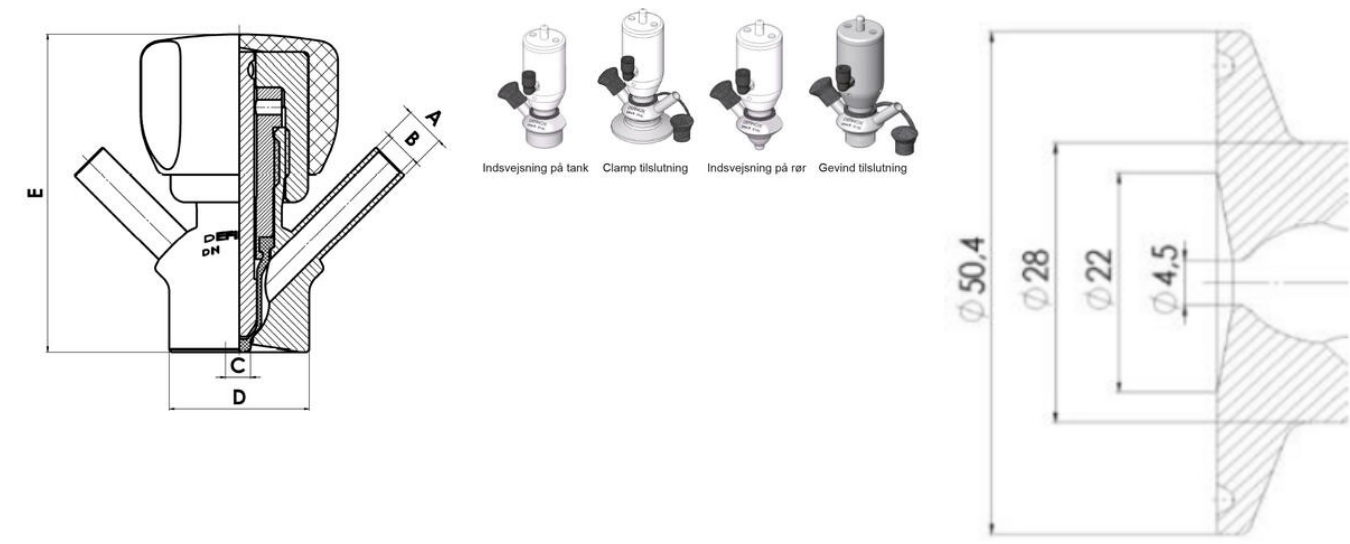
Clamp Ø 50,4
