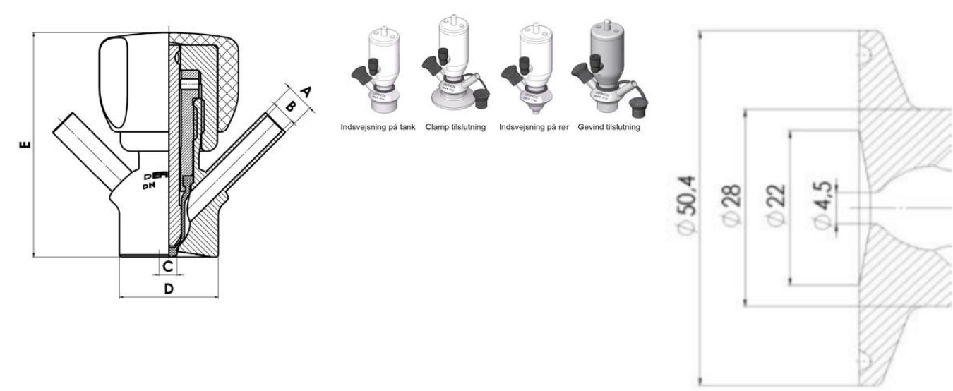
Clamp Ø 50,4
