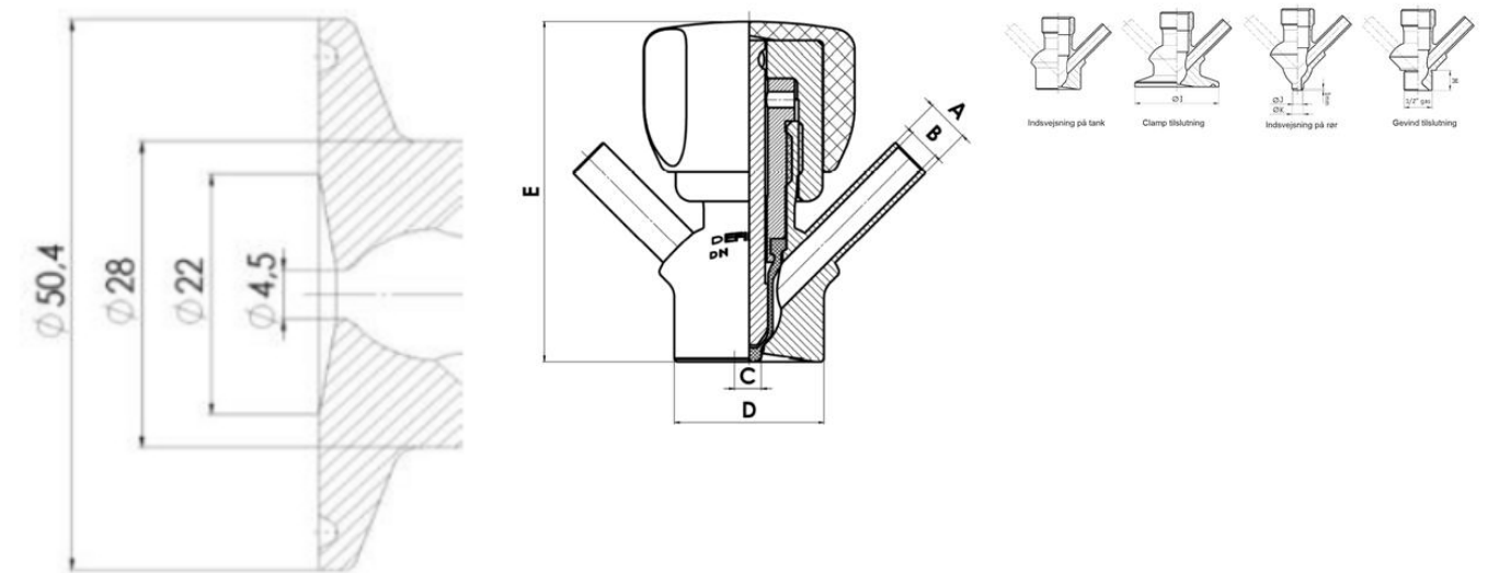
Clamp Ø 50,4
