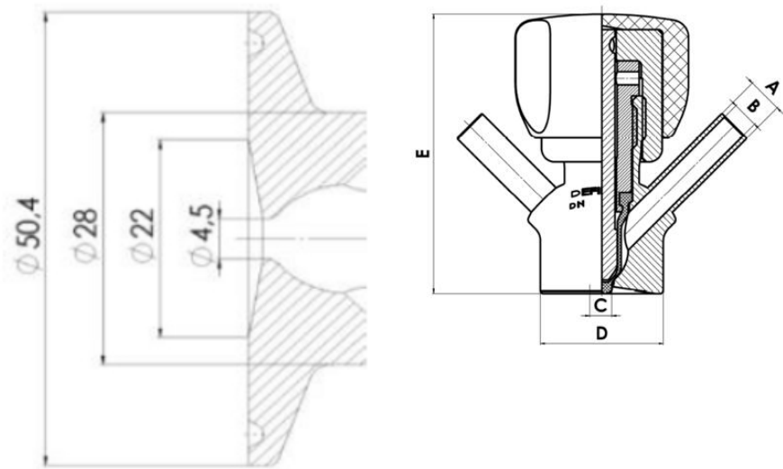
Clamp Ø 50,4
