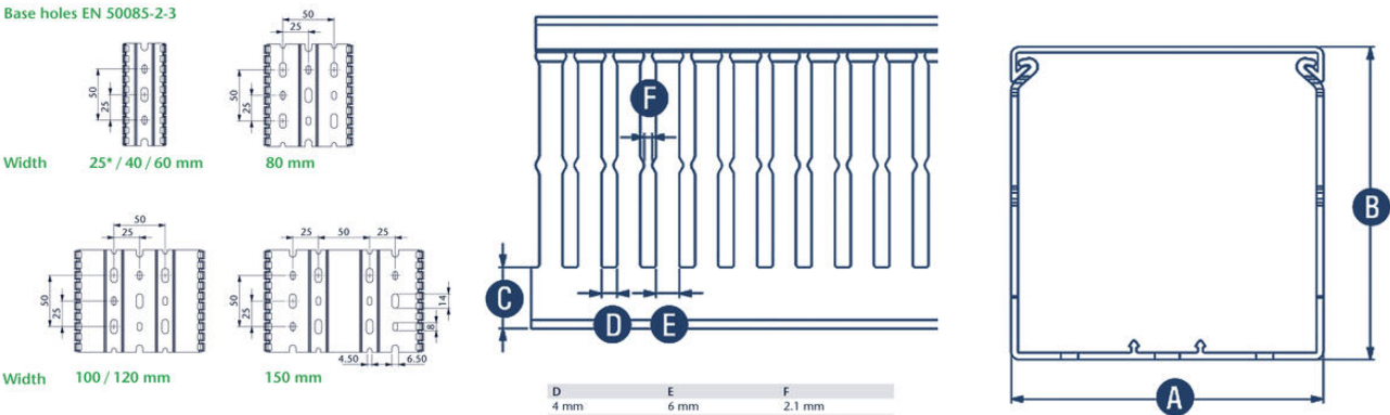
Base holes EN 50085-2-3
