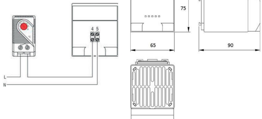
Thermostat KTO011 Heater CS(L) 028
