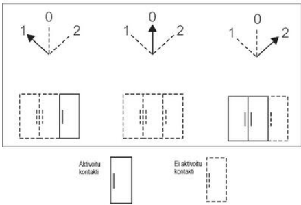
Kontaktien toiminta 3-asentoisille valintakytkimille (ei valoa) Valintakytkimen asento paneelin edestä katsottuna Kosketinyksiköiden toiminta paneelin edestä katsottuna
