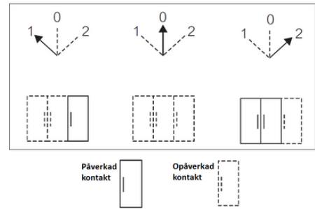
Kontakternas funktion till obelyst vred med 3 positioner Vredets position sett framifrån panelen. Kontaktblockens aktivitet sett framifrån panelen.
