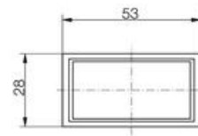
Håltagning med frontram 25x50 mm
