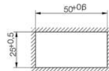
Håltagning med frontram 25x50 mm
